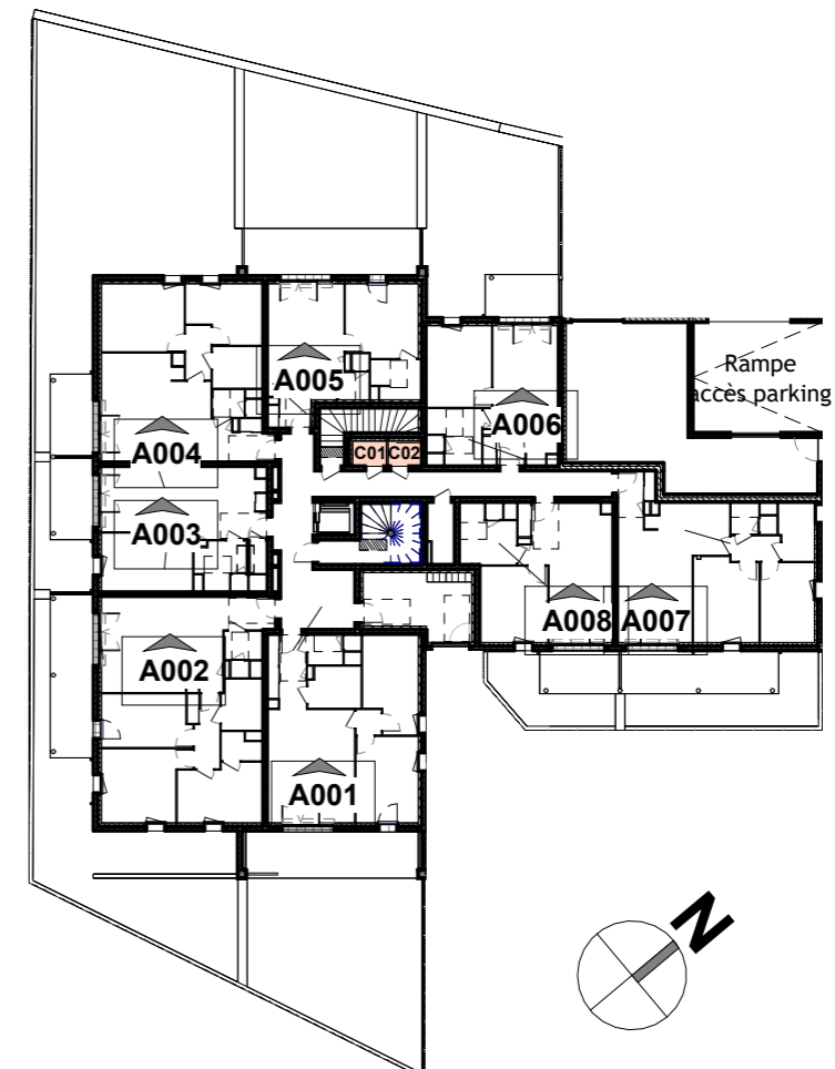
PLAN DE REPERAGE DES CELLIERS - PLAN RDC
