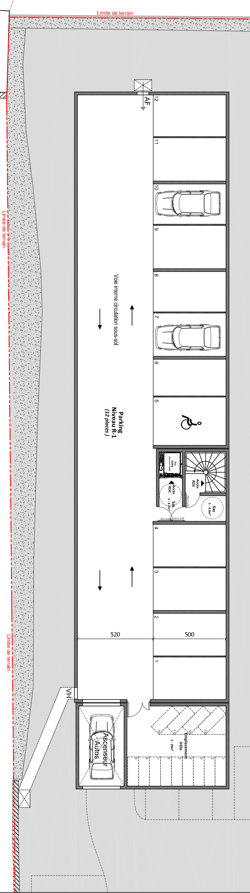
Plan du sous-sol R-1 Ech. 1/150e
