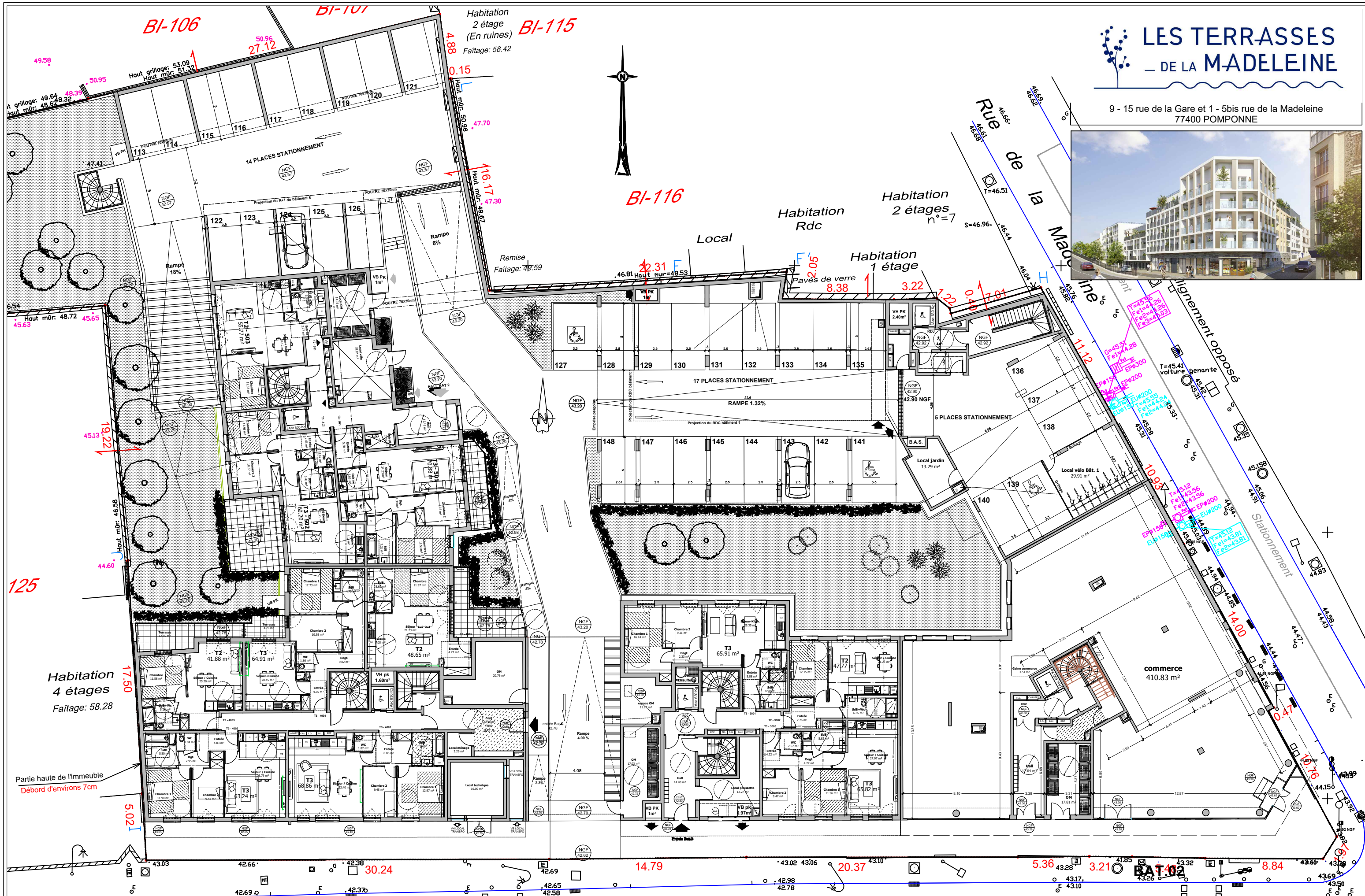
PLAN DU REZ DE CHAUSSEE
