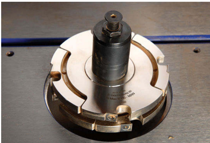
Tenonneuse équipée de deux plateaux à tenonner. L'utilisation de deux plateaux permet de réaliser des tenons précis en une seule passe.
