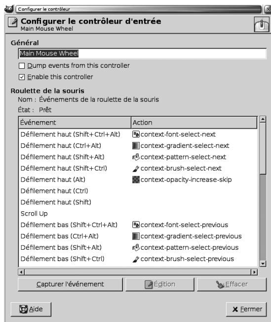
FIGURE A-4 Raccourcis souris et touches de direction
