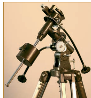
Une monture équatoriale motorisable. En l'absence de moteur, à cause des vibrations et des irrégularités produites, les mouvements manuels peuvent seulement être employés pour recentrer la planète et non pour assurer son suivi continu.
