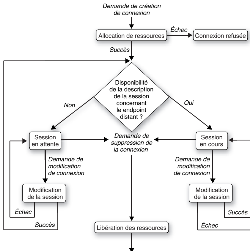
Figure 5.6 Diagramme d'états d'une passerelle
