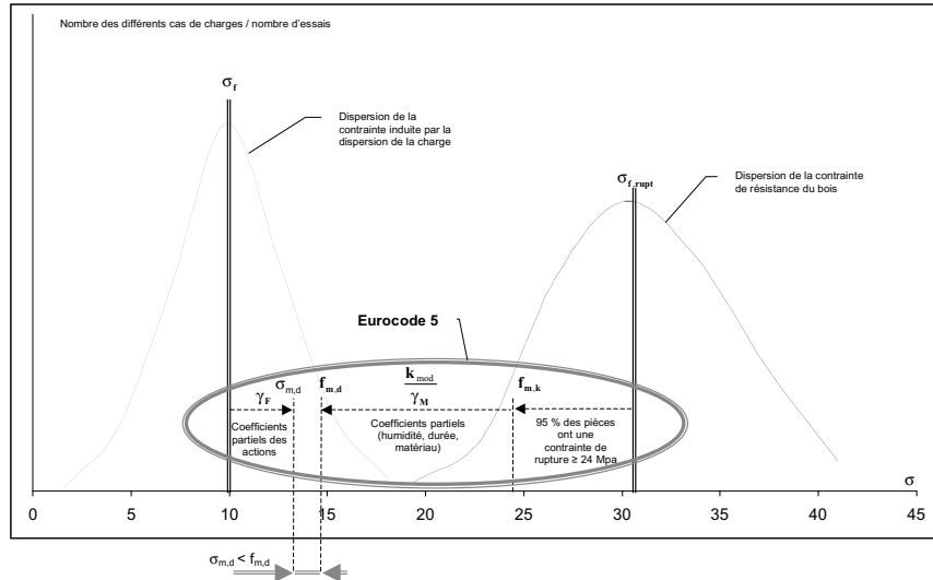
Schéma 10 : principes de justification des états limites ultimes des eurocodes 5, vérifications de la contrainte de flexion
