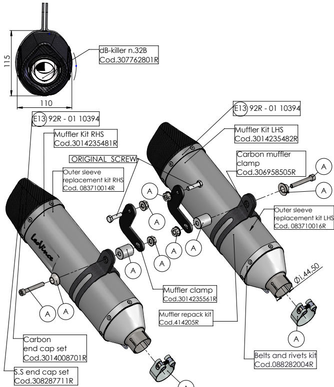
ART. 14235E SPARE PARTS
