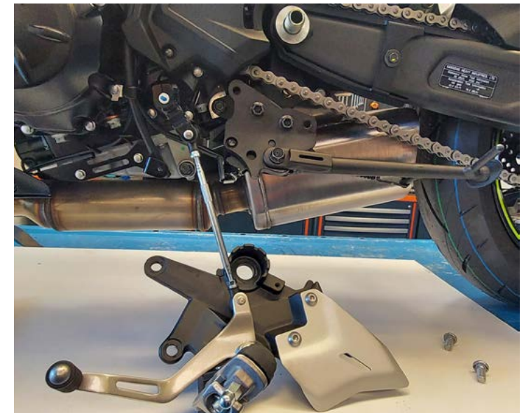
PHOTO 8 (KAWASAKY NINJA 650)
