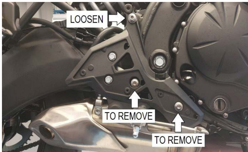
PHOTO 1 (KAWASAKY VERSYS 650)
