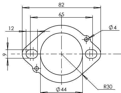
Flange kit Cod.204569R
