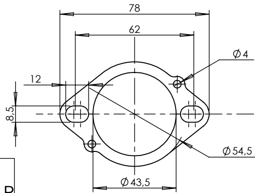
Flange cod.204448
