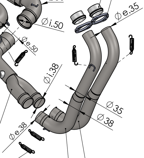
2x Flange cod.204569
